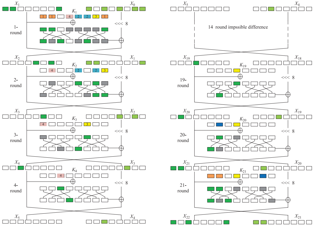
图2 21轮LBlock-s的不可能差分分析 (前面加4轮, 后面加3轮)
