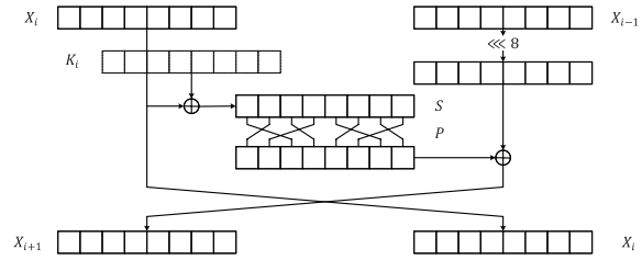
图1 LBlock-s算法中的轮函数
